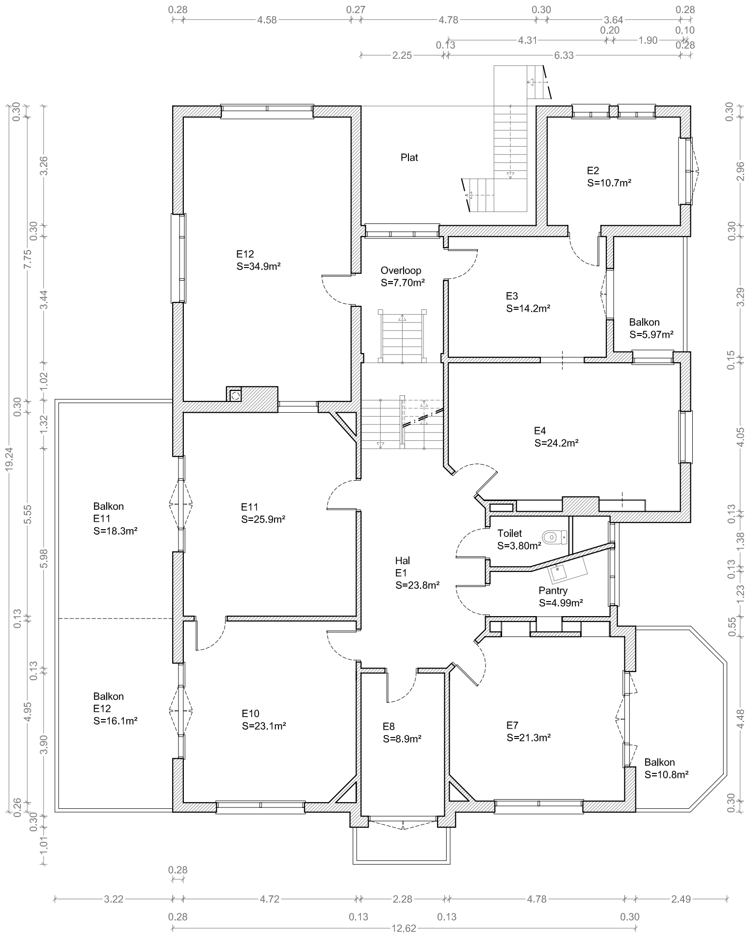
VILLA KLEIN DREIJEN_e:1/100_160627 1e Verdieping TOTAAL GBO=237.50m 2
